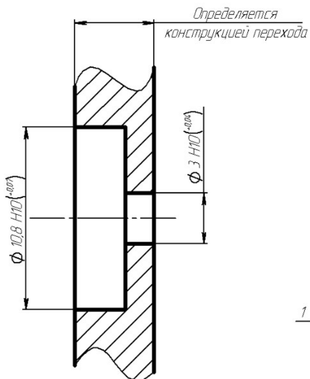
Отверстие в приборной панели
